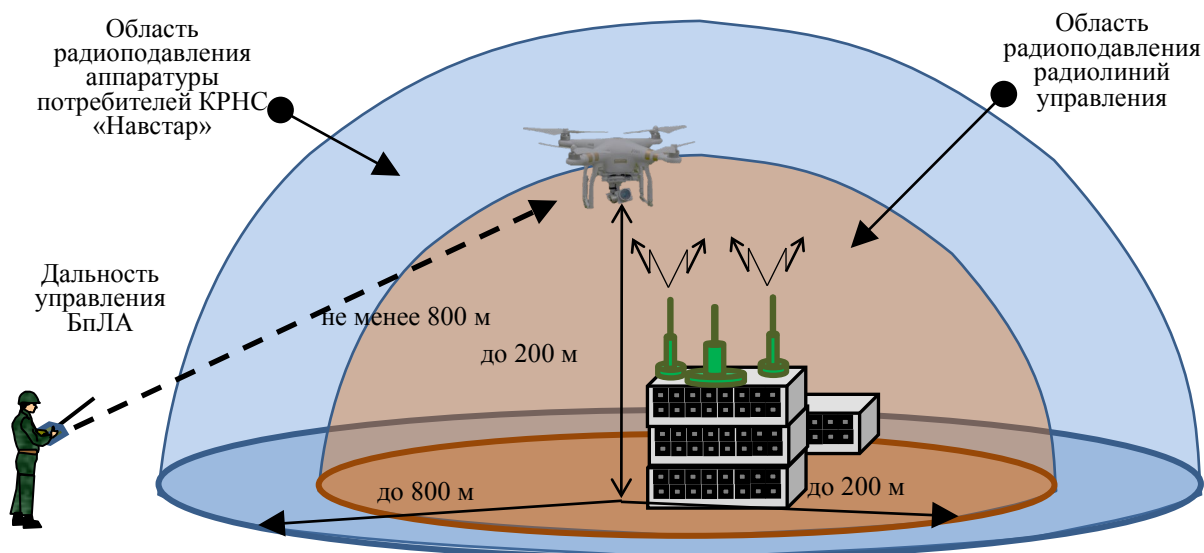
Рис. 13. Вариант применения станции помех РП-377УВМ1Л «Лесочек», при РЭП радиопередачи управления и аппаратуры потребителя КРНС БПЛА
